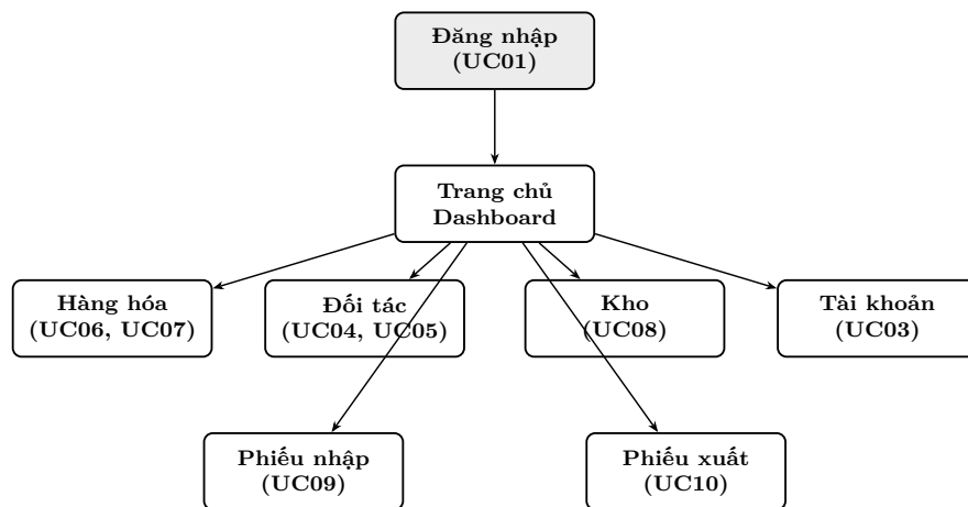
Figure 1: Sơ đồ điều hướng màn hình chính (theo use case)
